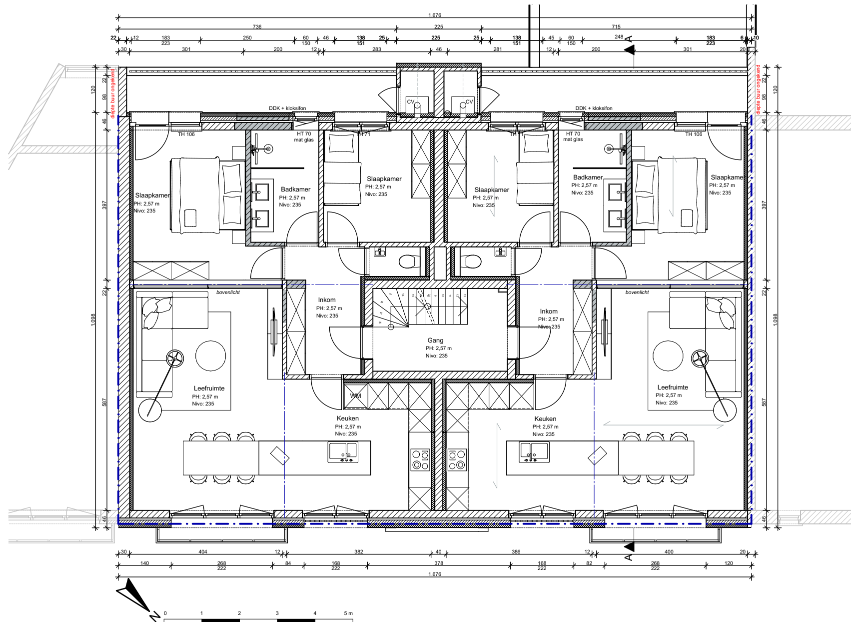
Verdieping 1 NT
